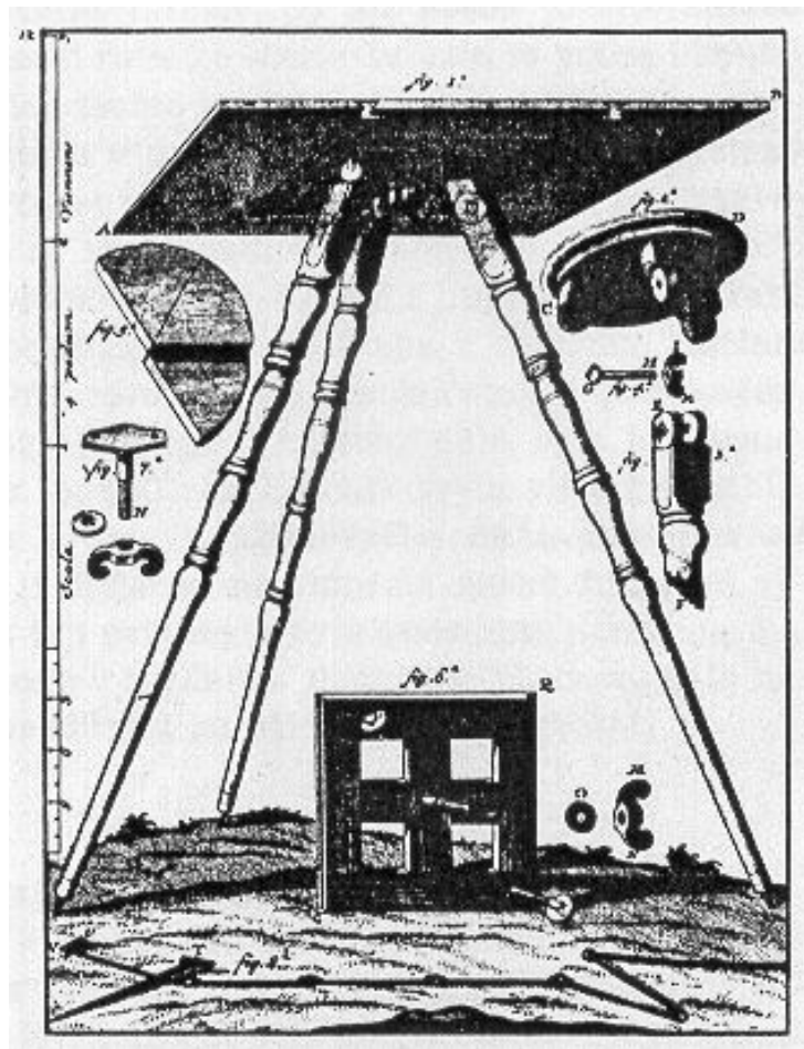
Obr. 13 - měřický stůl starého typu (konec 18. století), [37]
