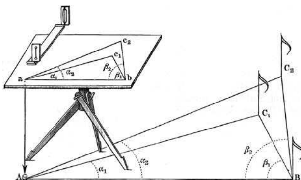
Obr. 12 – měřický stůl, [4]
