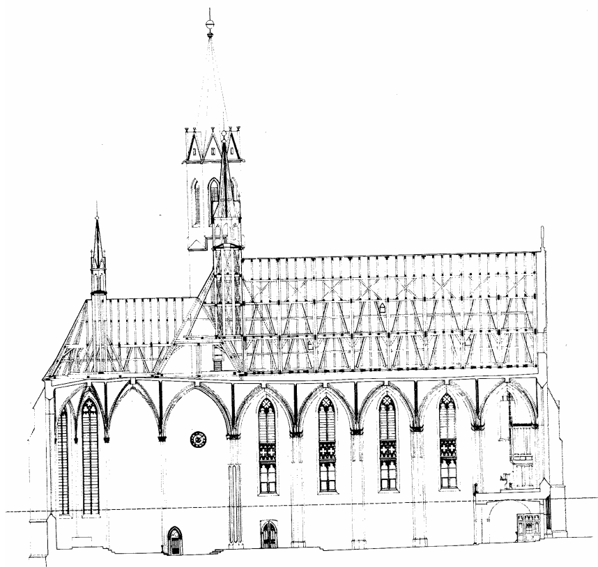
Vyšší Brod, klášterní kostel, podélný řez
