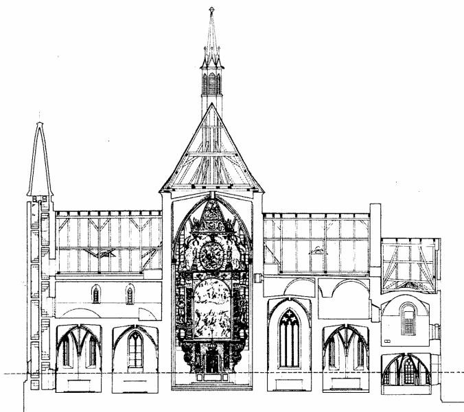
Vyšší Brod, klášterní kostel, příčný řez
