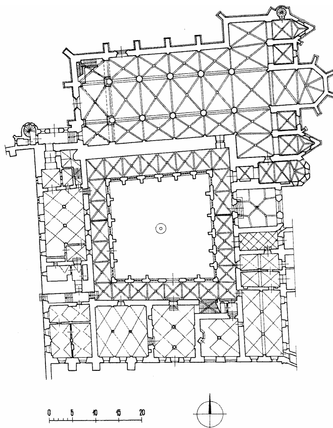
Půdorys kláštera, kostela a křížové chodby ve Vyšším Brodě
