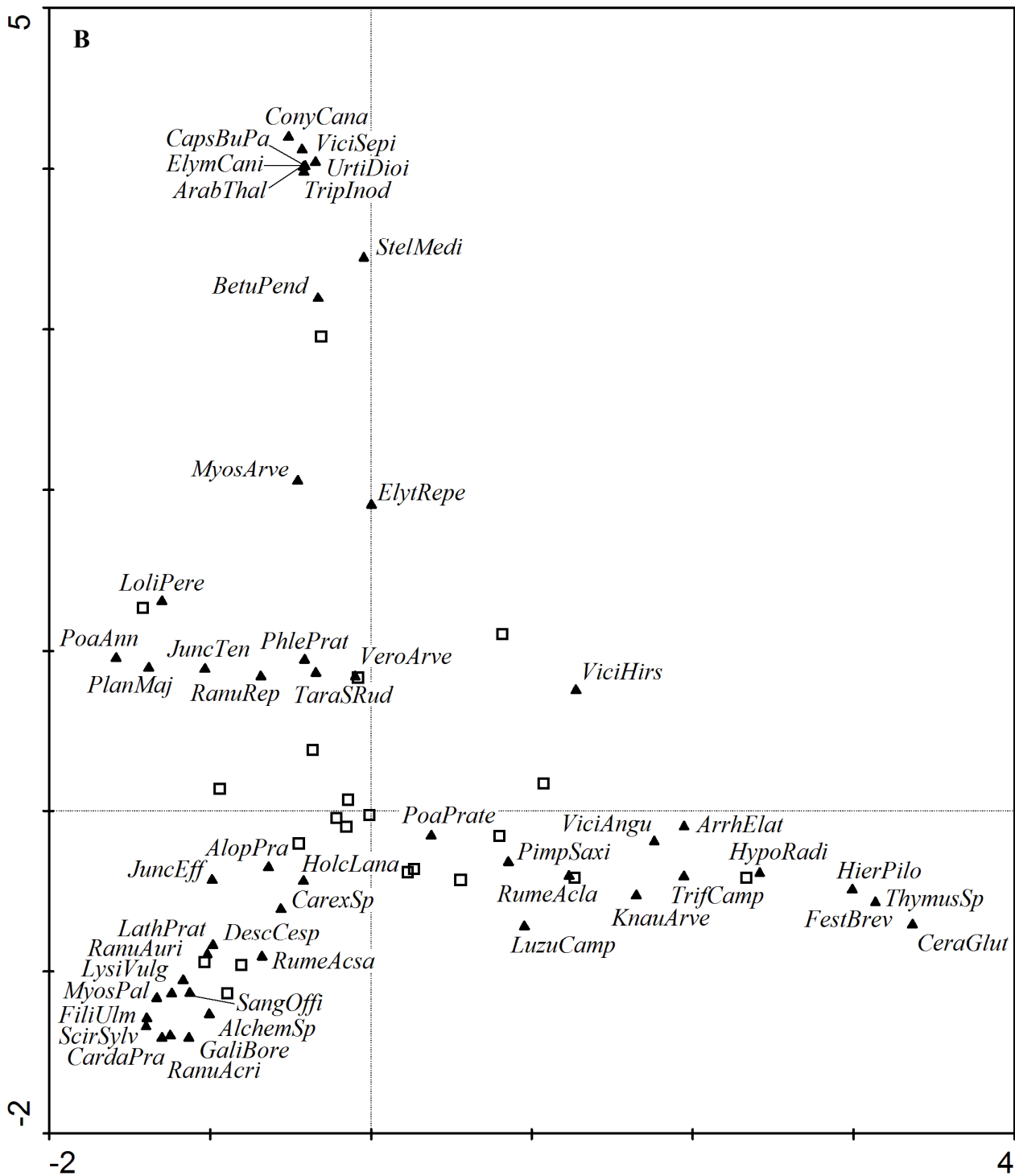
Obrázek 7 (pokračování): ... LathPrat – Lathyrus pratensis , LoliPere – Lolium perenne , LuzuCamp – Luzula campestris , LysiVulg – Lysimachia vulgaris , MyosArve – Myosotis arvensis , MyosPal – Myosotis palustris , PhlePrat – Phleum pratense , PimpSaxi – Pimpinella saxifraga , PlanMaj – Plantago major , PoaAnn – Poa annua , PoaPrate – Poa pratensis , RanuAcri – Ranunculus acris , RanuAuri – R. auricomus , RanuRep – R. repens , RumeAcla – Rumex acetosella , RumeAcsa – R. acetosa , SangOffi – Sanguisorba officinalis , ScirSylv – Scirpus sylvaticus , StelMedi – Stellaria media , TaraSRud – Taraxacum sect. Ruderalia , ThymusSp – Thymus sp. , TrifCamp – Trifolium campestre , TripInod – Tripleurospermum inodorum , UrtiDioi – Urtica dioica , VeroArve – Veronica arvensis , ViciAngu – Vicia angustifolia , ViciHirs – V. hirsuta , ViciSepi – V. sepium ).
