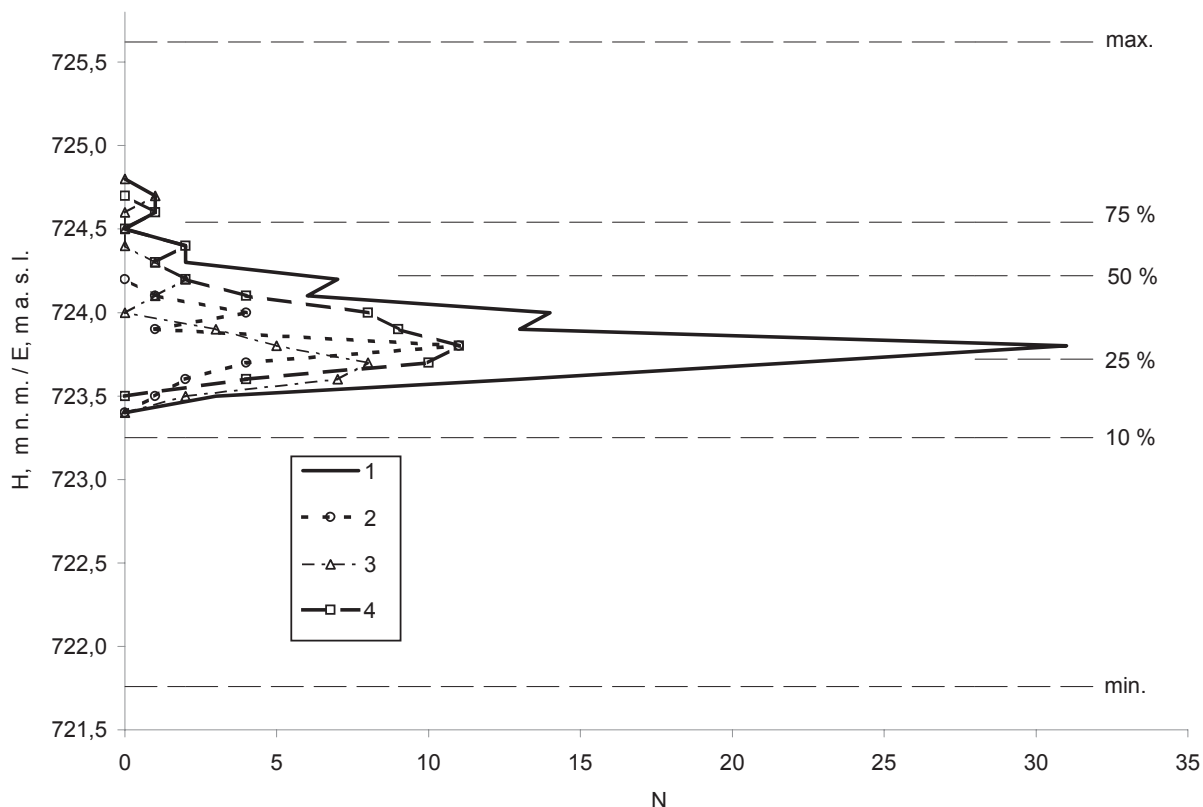
Obr. 6. Histogram četnosti minimální nadmořské výšky výskytu kořenicích makrofyt na lokalitách v litorálu nádrže Lipno. Vodorovné čáry vyznačují: maximum, vybrané procentily (75 %, 50 %, 25 %, 10 %) a minimum hodnot výšky vodní hladiny v nádrži v souboru denních dat 1991–2005. Legenda: 1 – všechny lokality; 2 – zátoky; 3 – lokality s přítoky; 4 – otevřené lokality.
