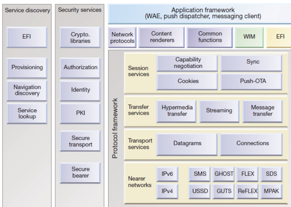
Obrázek 3 – Vrstvy WAP architektury
