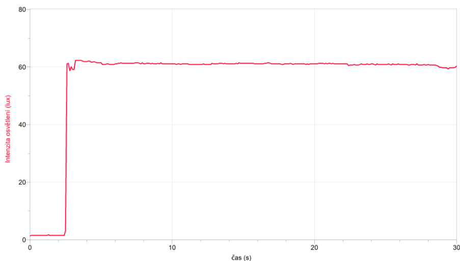
Graf 9.16.2: Graf náběhu klasické žárovky Tes - lamps 60 W na plný výkon
