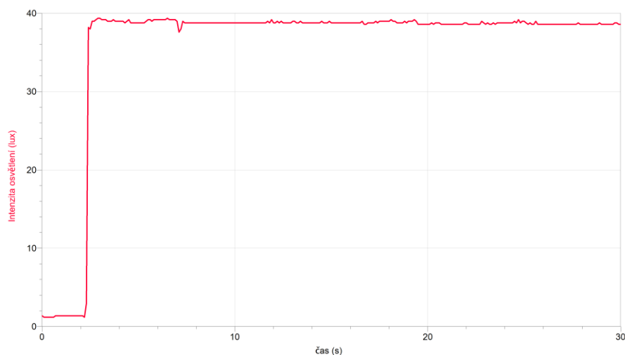
Graf 9.13.2: Graf náběhu klasické žárovky NBB Bohemia 40 W na plný výkon
