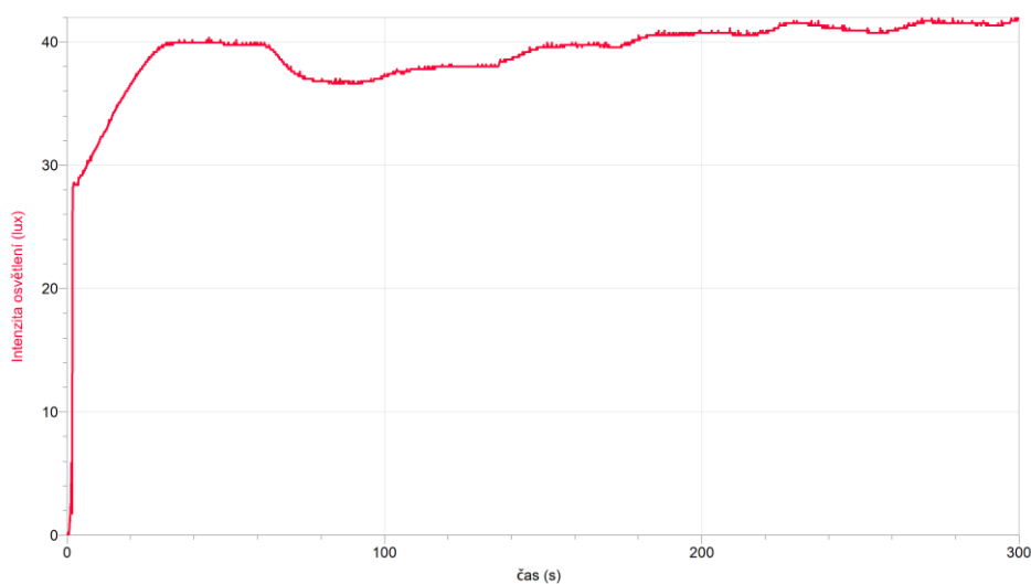
Graf 9.17.2: Graf náběhu kompaktní zářivky Konnoc 11 W na plný výkon
