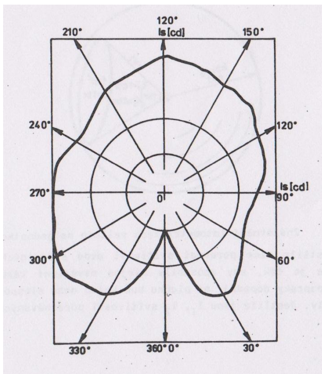
Obrázek 7.2: Vyzařovací diagram tvaru symetrické srdcovky
