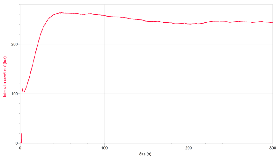
Graf 9.18.2: Graf náběhu kompaktní zářivky Eco lite 46 W na plný výkon
