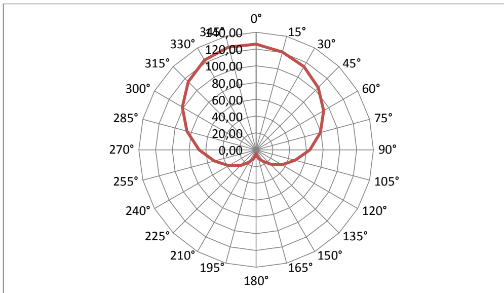
Graf 9.6.1: Vyzařovací diagram LED žárovky 10 W.
