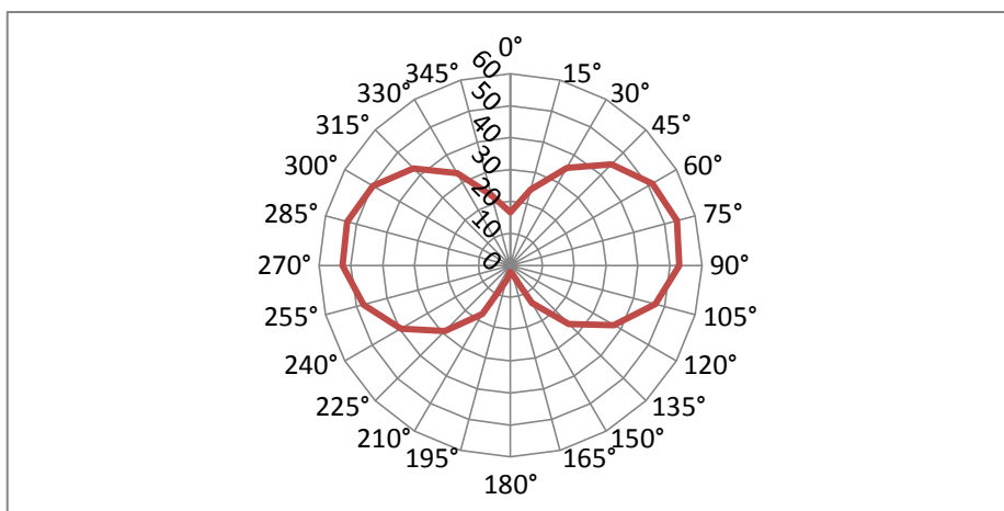
Graf 9.17.1: Vyzařovací diagram kompaktní zářivky Konnoc 11 W
