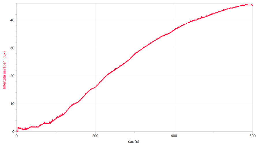
Graf 9.19.2: Graf náběhu kompaktní zářivky Hallux 8 W na plný výkon
