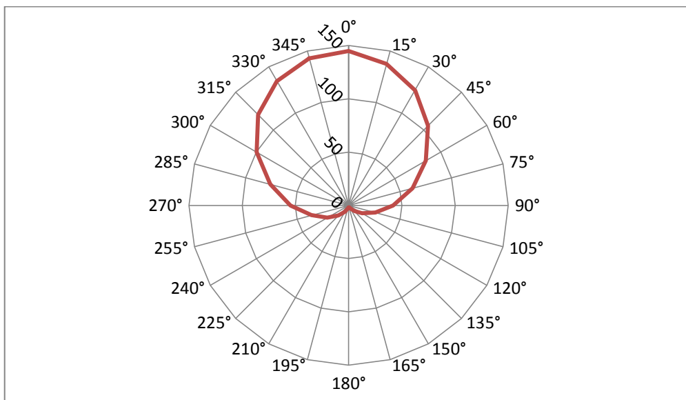
Graf 9.1.1: Vyzařovací diagram LED žárovky BL1 9 W
