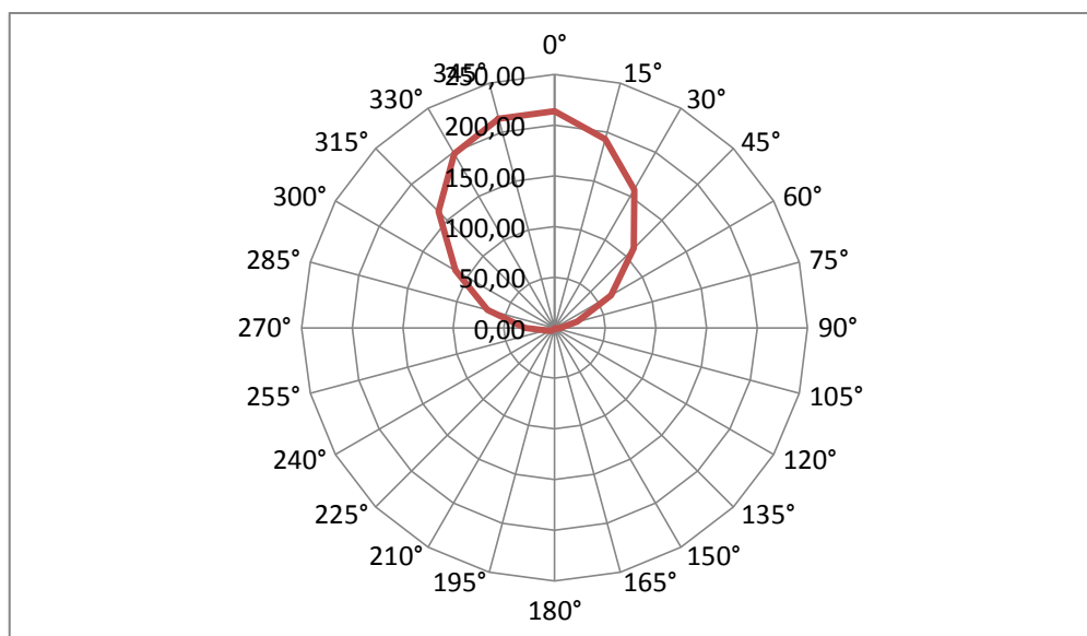
Graf 9.9.1: Vyzařovací diagram LED žárovky 3 W.
