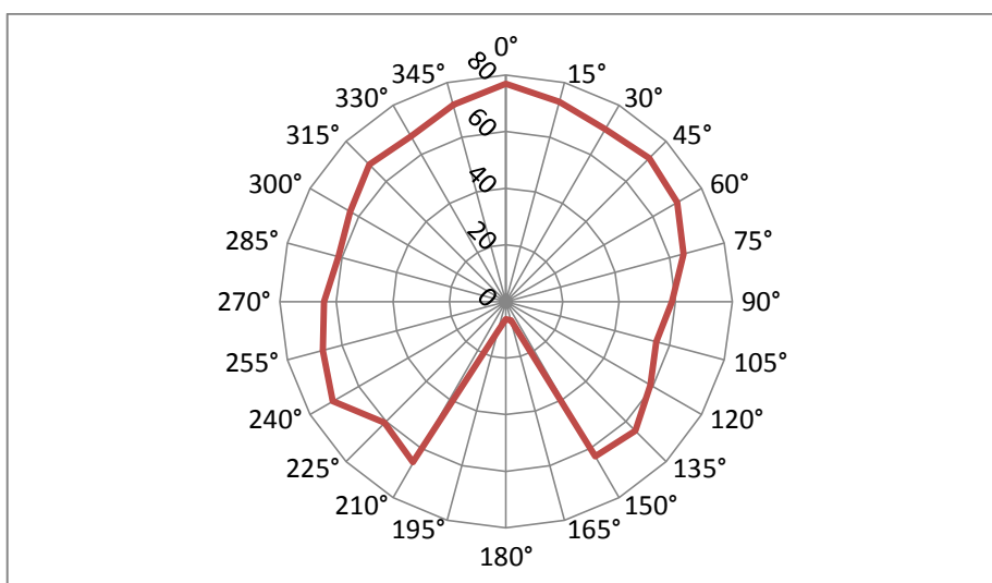
Graf 9.16.1: Vyzařovací diagram klasické žárovky Tes - lamps 60 W
