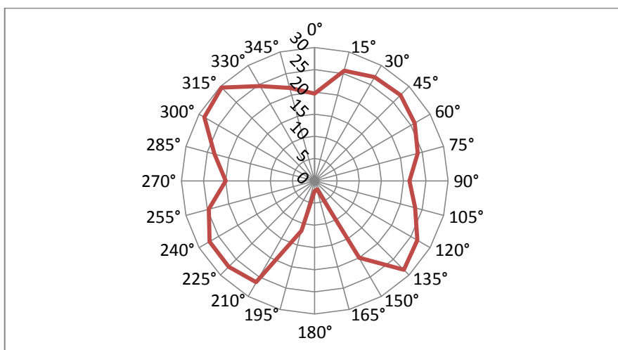
Graf 9.13.1: Vyzařovací diagram klasické žárovky NBB Bohemia 40 W
