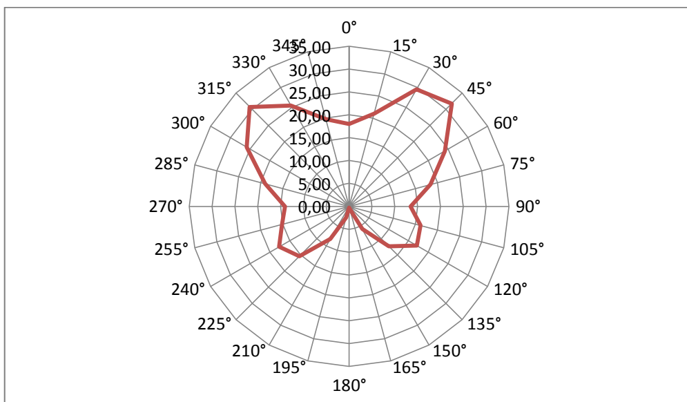
Graf 9.7.1: Vyzařovací diagram LED žárovky 3 W.
