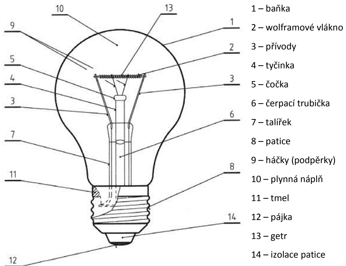
Obrázek 3.1: Konstrukce klasické žárovky [8]
