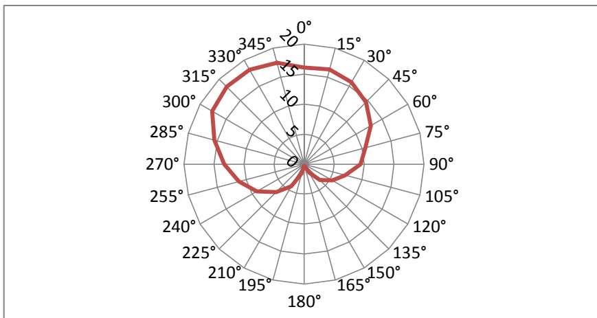
Graf 9.19.1: Vyzařovací diagram kompaktní zářivky Hallux 8 W
