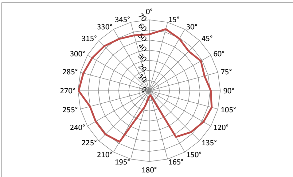
Graf 9.14.1: Vyzařovací diagram klasické žárovky Radium 60 W
