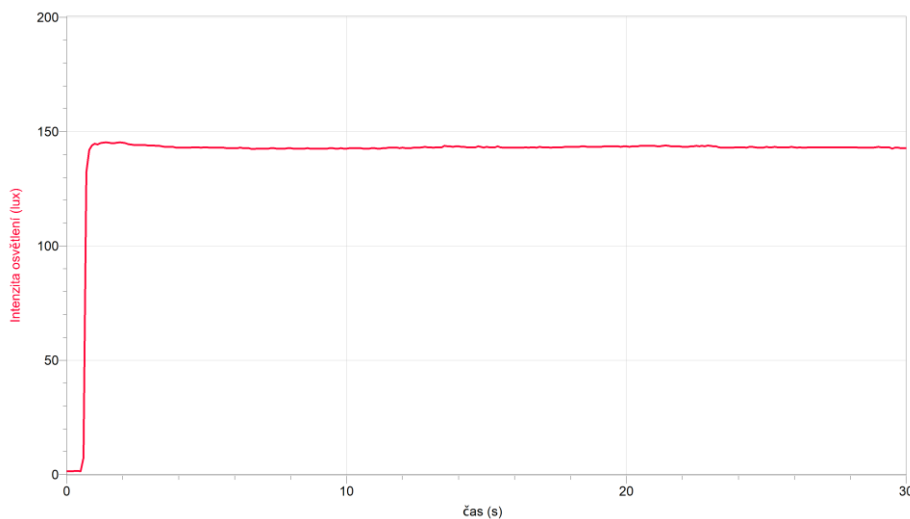
Graf 9.12.2: Graf náběhu klasické mléčné žárovky Novaline 100 W na plný výkon
