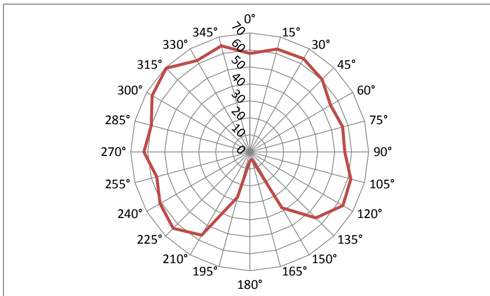
Graf 9.11.1: Vyzařovací diagram klasické žárovky NBB Bohemia 75 W
