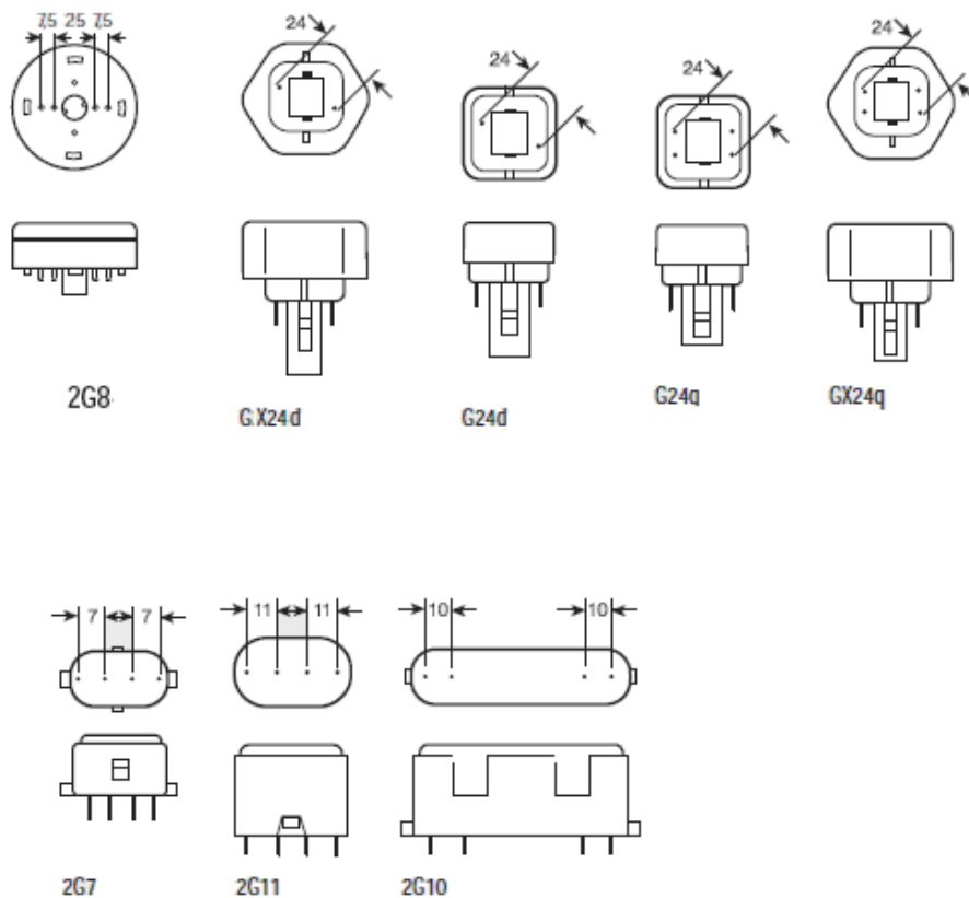
Obrázek 4.2: patice 2G8, GX24d, G24d, G24q, GX24q, 2G7, 2G11, 2G10
