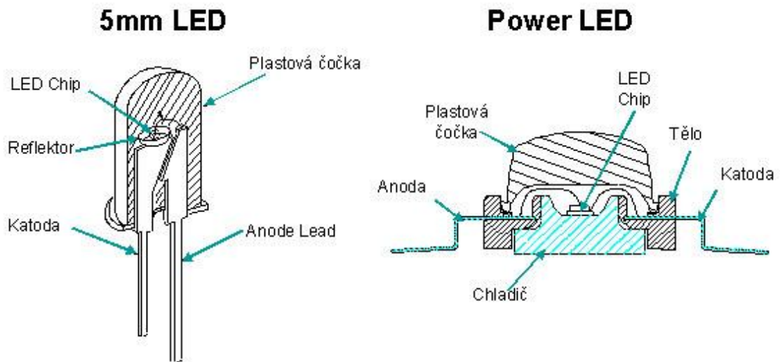
Obrázek 6.1: Konstrukce LED [24]
