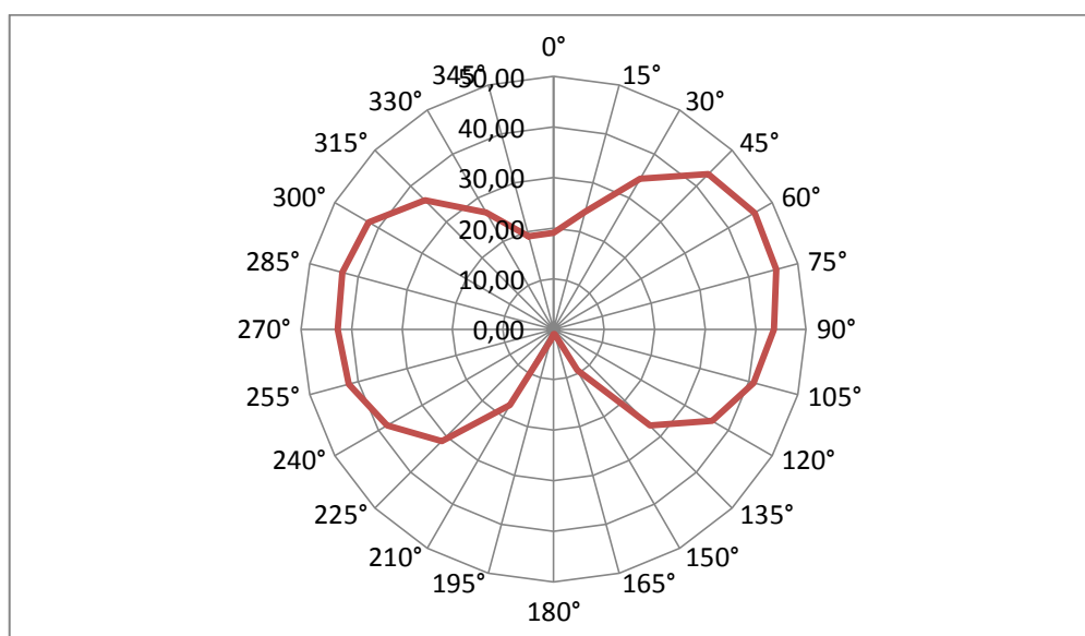
Graf 9.8.1: Vyzařovací diagram LED žárovky 4 W.
