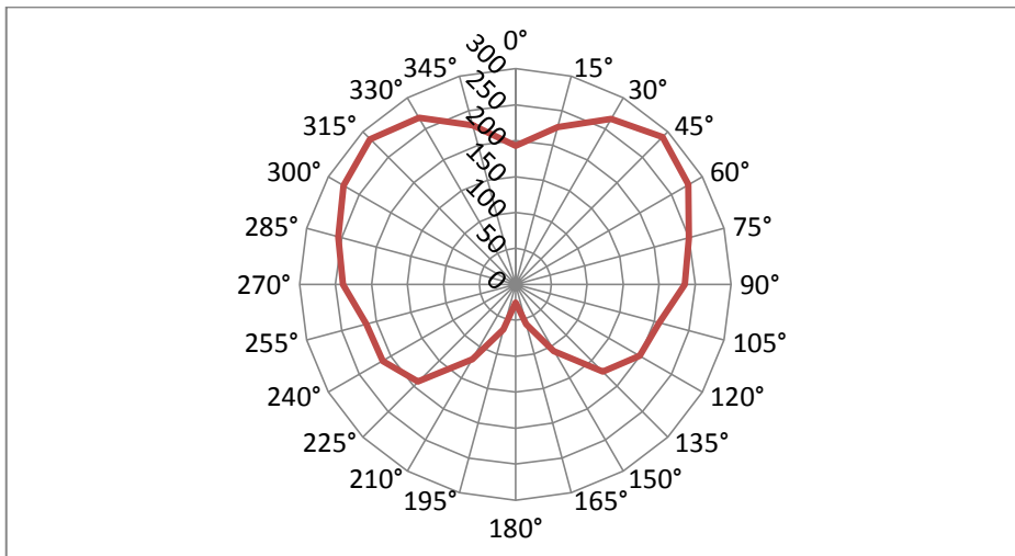
Graf 9.18.1: Vyzařovací diagram kompaktní zářivky Eco lite 46 W
