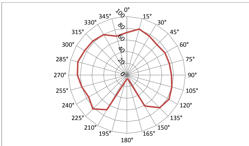
Graf 9.10.1: Vyzařovací diagram klasické žárovky Osram 75 W
