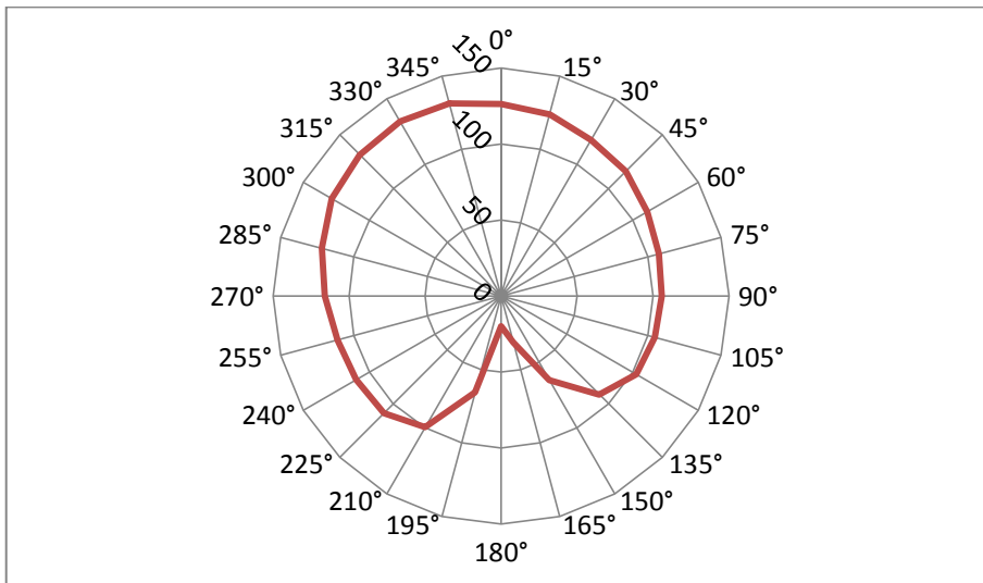
Graf 9.12.1: Vyzařovací diagram klasické mléčné žárovky Novaline 100 W
