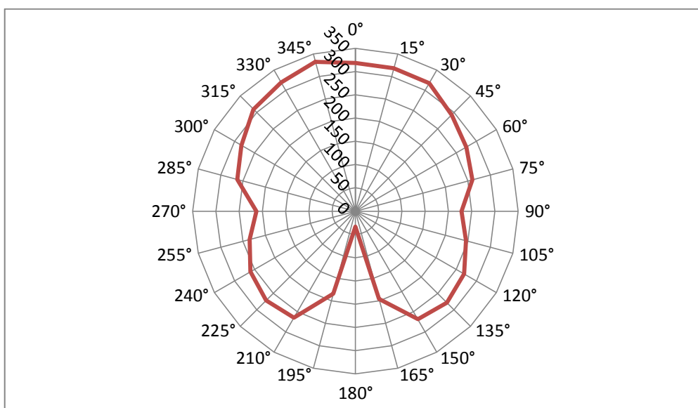
Graf 9.15.1: Vyzařovací diagram klasické žárovky 200 W
