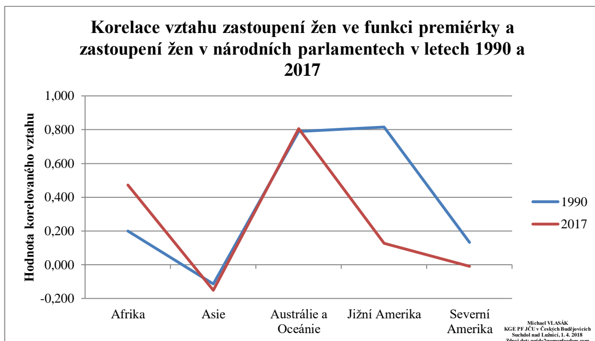
Graf č. 5: Korelace vztahu zastoupení žen ve funkci premiérky a zastoupení žen v národních parlamentech v letech 1990 a 2017
