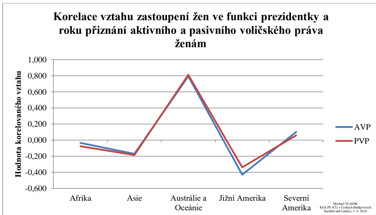
Graf č. 4: Korelace vztahu zastoupení žen ve funkci prezidentky a roku přiznání aktivního a pasivního voličského práva ženám
