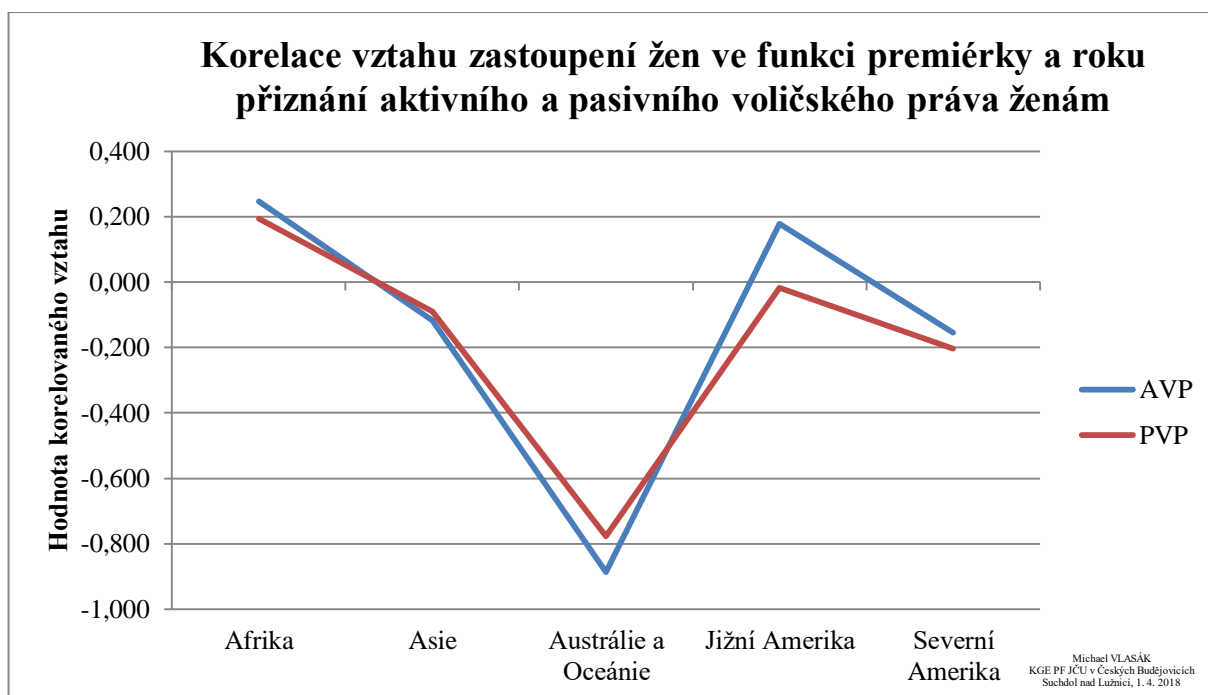
Graf č. 8: Korelace vztahu zastoupení žen ve funkci premiérky a roku přiznání aktivního a pasivního volečského práva ženám
