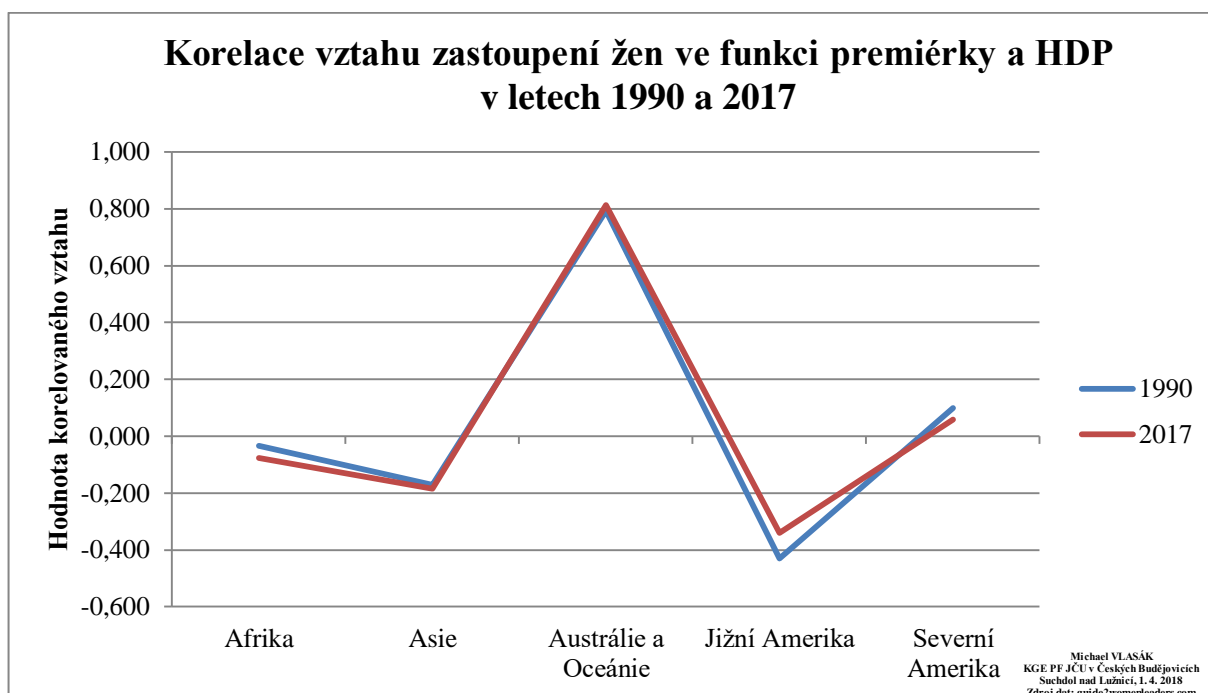
Graf č. 7: Korelace vztahu zastoupení žen ve funkci premiérky a HDP v letech 1990 a 2017
