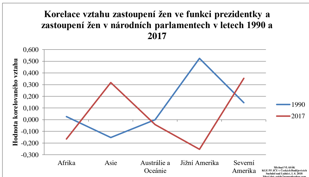
Graf č. 1: Korelace vztahu zastoupení žen ve funkci prezidentky a zastoupení žen v národních parlamentech v letech 1990 a 2017
