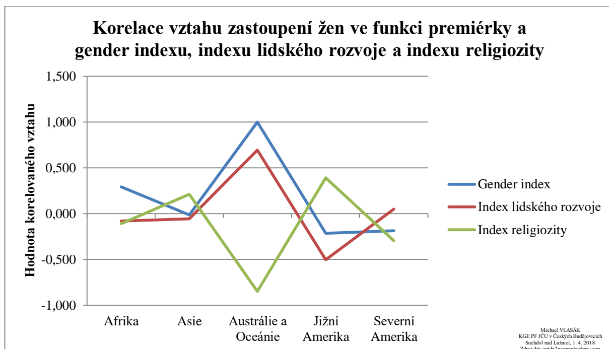
Graf č. 6: Korelace vztahu zastoupení žen ve funkci premiérky a gender indexu, indexu lidského rozvoje a indexu religiozity
