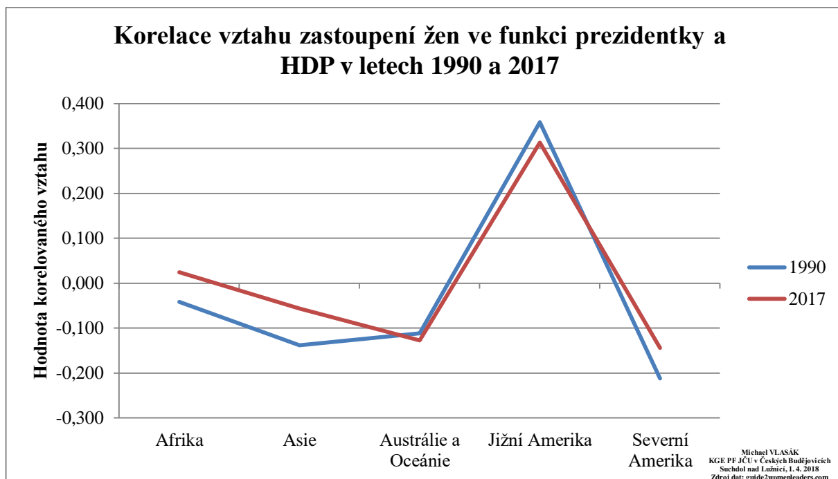
Graf č. 3: Korelace vztahu zastoupení žen ve funkci prezidentky a HDP v letech 1990 a 2017
