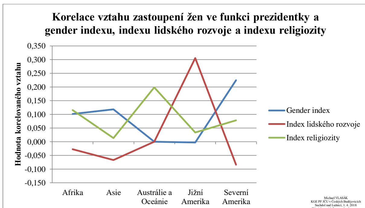
Graf č. 2: Korelace vztahu zastoupení žen ve funkci prezidentky a gender indexu, indexu lidského rozvoje a indexu religiozity
