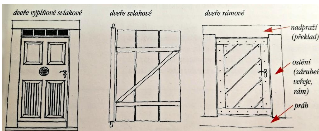
Obrázek 8 - Typy dveří (Zdroj: David, Soukup, 200)
