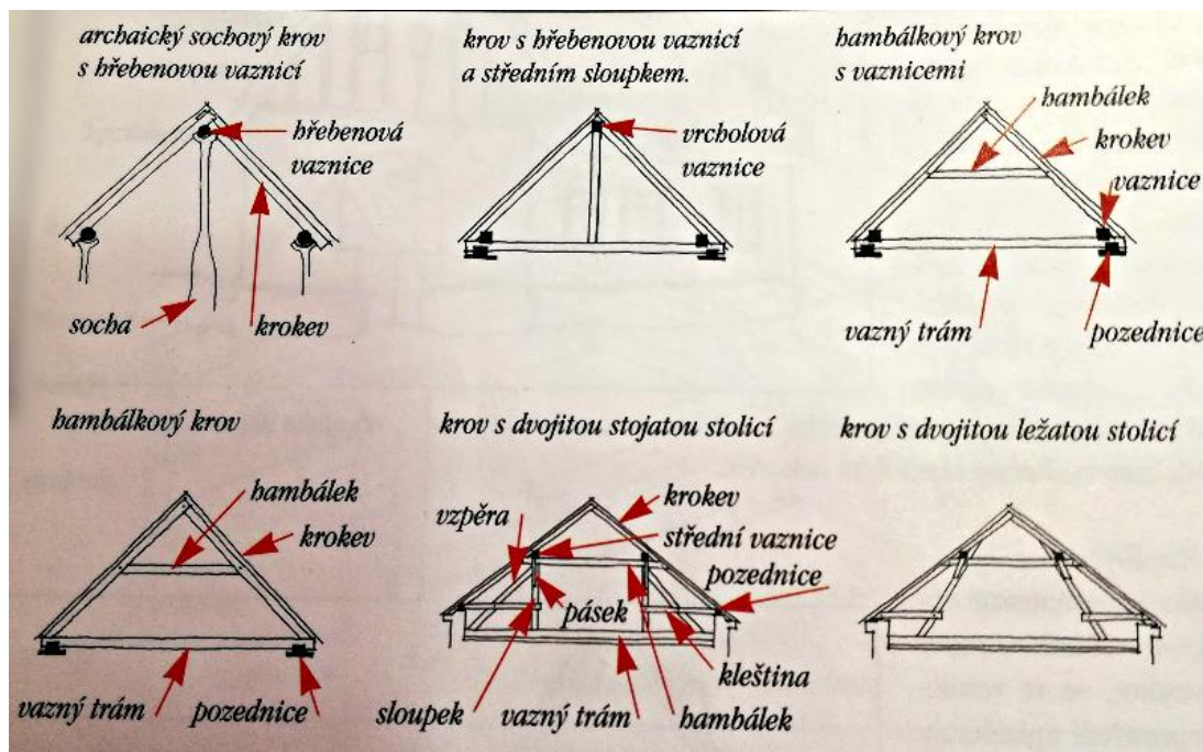
Obrázek 6 - Příklady krovů (Zdroj: David, Soukup, 2000)
