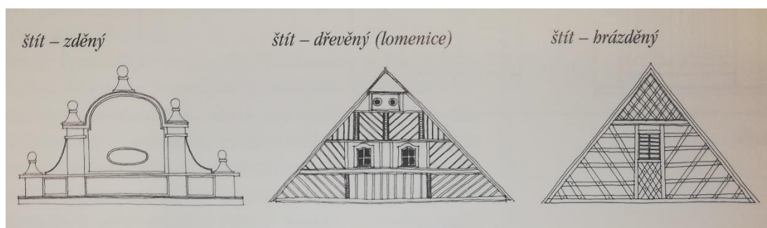
Obrázek 10 - Typy štítů (Zdroj: David, Soukup, 2000)
