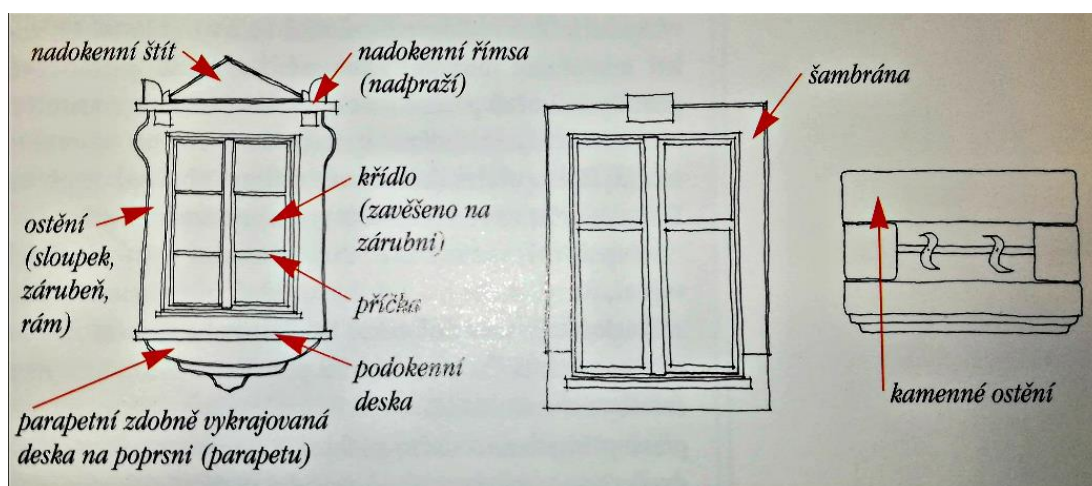
Obrázek 9 - Okna v lidové architektuře (Zdroj: David, Soukup, 2000)
