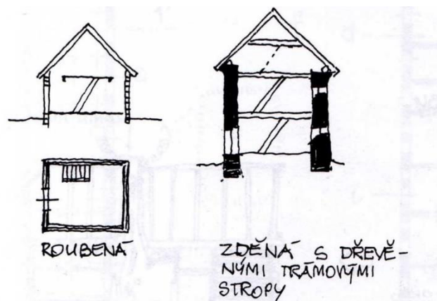
Obrázek 12 - Schémata řešení sýpek (Zdroj: Sýkora, 1998)
