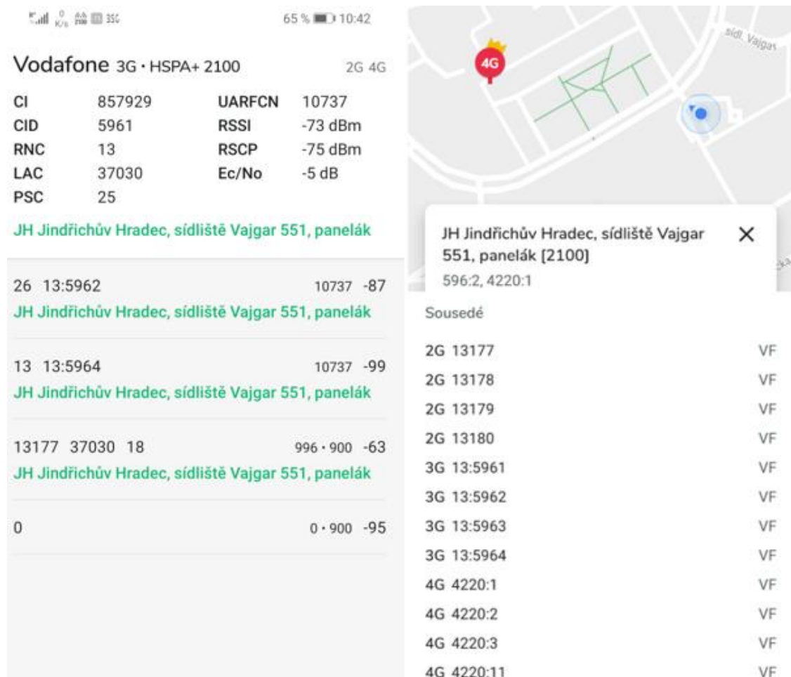
Obrázek 32: Měření signálu 3G (zdroj: vlastní výzkum)
