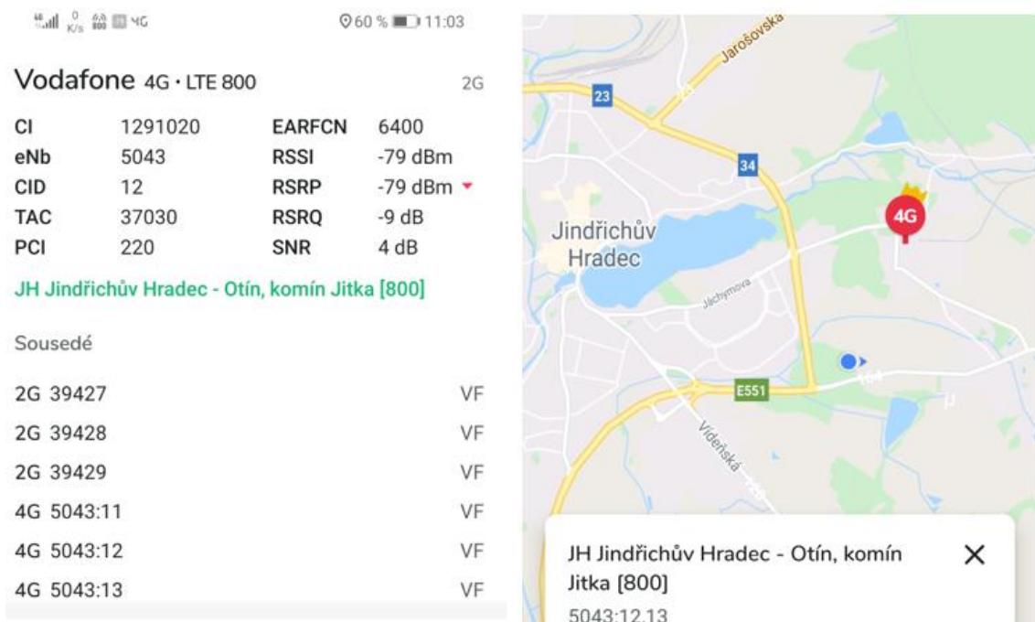
Obrázek 34: Měření signálu (zdroj: vlastní výzkum)
