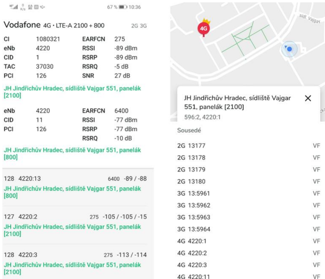
Obrázek 30: Měření signálu (zdroj: vlastní výzkum)
