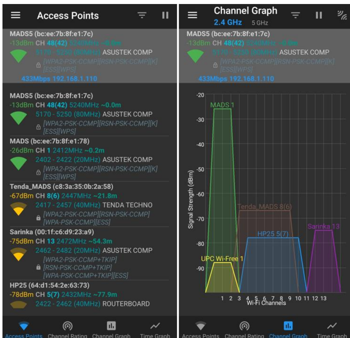
Obrázek 41: Optimalizace wifi signálu (zdroj: vlastní výzkum)
