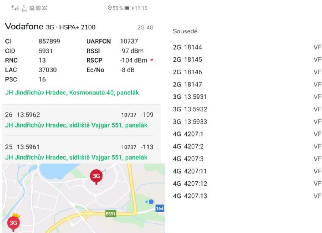
Obrázek 37: Měření signálu (zdroj: vlastní výzkum)
