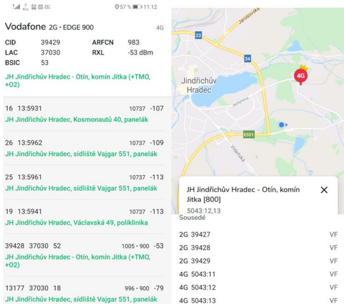
Obrázek 35: Měření signálu (zdroj: vlastní výzkum)
