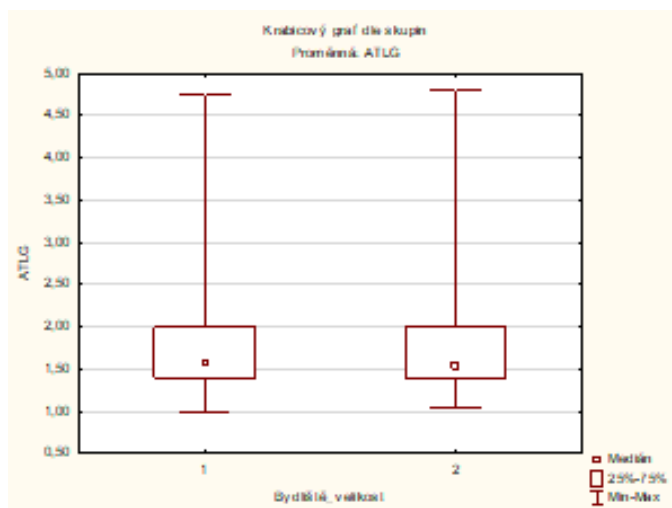
Graf 6: Krabicový graf pro H_3 (1=do 20tis.obyvateľ; 2=nad 20tis.obyvateľ)
