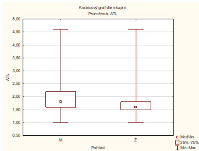
Graf 3: Krabicový graf pro H_1 (ATL) (M=muži; Z=ženy)
