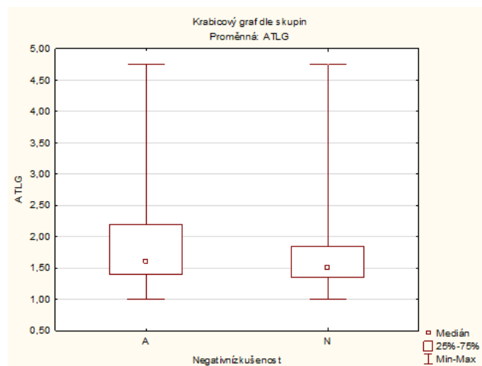
Graf 14: Krabicový graf pro H_{11}(A=ano;N=ne)
