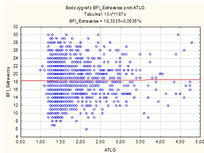
Graf 8: Graf Spearmanovy korelace pro H_5 (Extravertze+ATLG)
