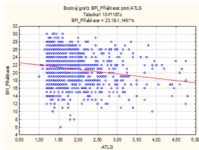
Graf 9: Graf Spearmanovy korelace pro H_6 (Přívětivost+ATLG)
