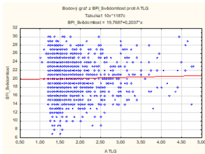
Graf 10: Graf Spearmanovy korelace pro H_7 (Svědomitost+ATLG)
