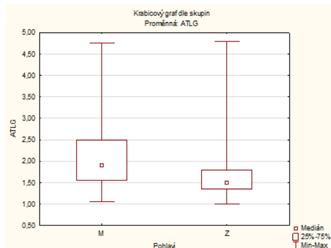
Graf 2: Krabicový graf pro H_1 (ATLG) (M=muži; Z=ženy)
