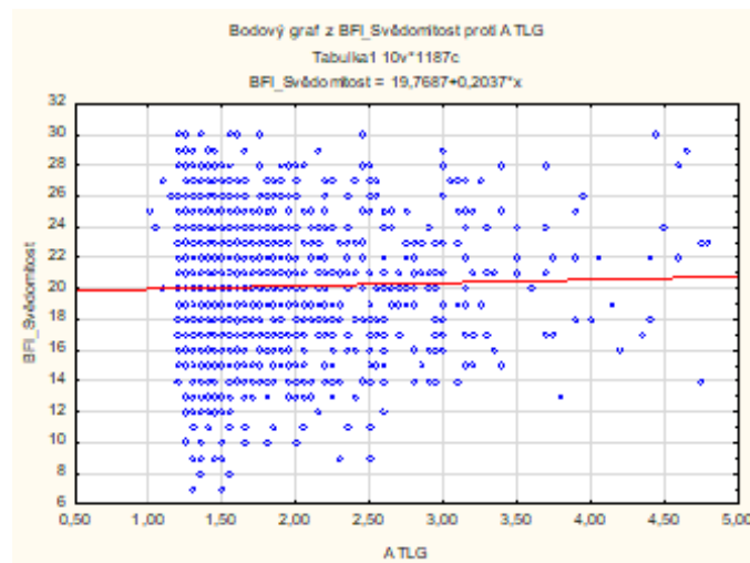
Graf 11: Graf Spearmanovy korelace pro H_8 (Negativní emocionalita+ATLG)
