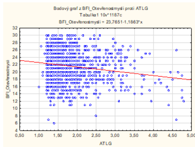
Graf 12: Graf Spearmanovy korelace pro H_9 (Otevřenost mysli+ATLG)
