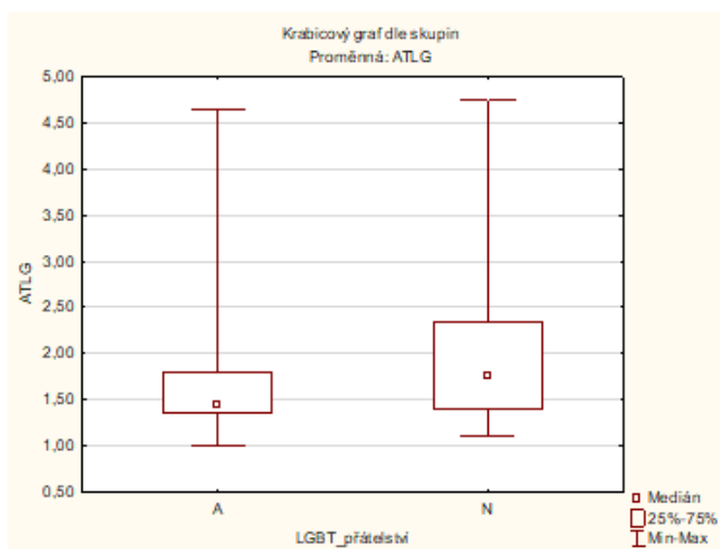
Graf 13: Krabicový graf pro H_{10} (A=ano;N=ne)
