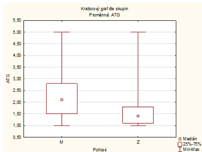
Graf 4: Krabicový graf pro H_1 (ATG) (M=muži; Z=ženy)
