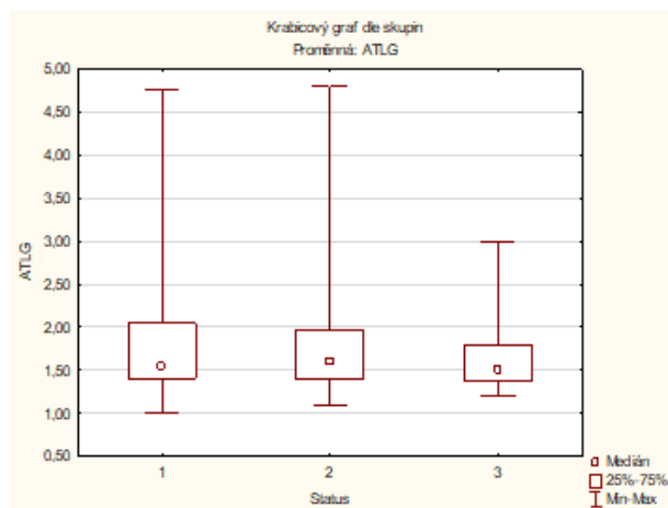
Graf 7: Krabicový graf pro H_4 (1=studenti; 2=pracující; 3=nepracující)
