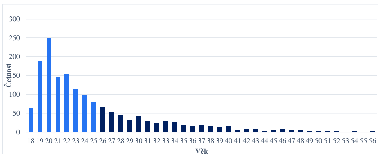
Graf 1: Četnost zastoupení v testovaném vzorku na základě věku
