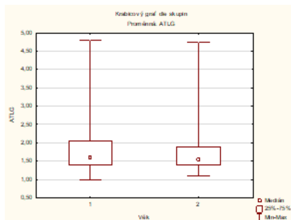
Graf 5: Krabicový graf pro H_2 (1=18-26 let; 2=27+ let)
