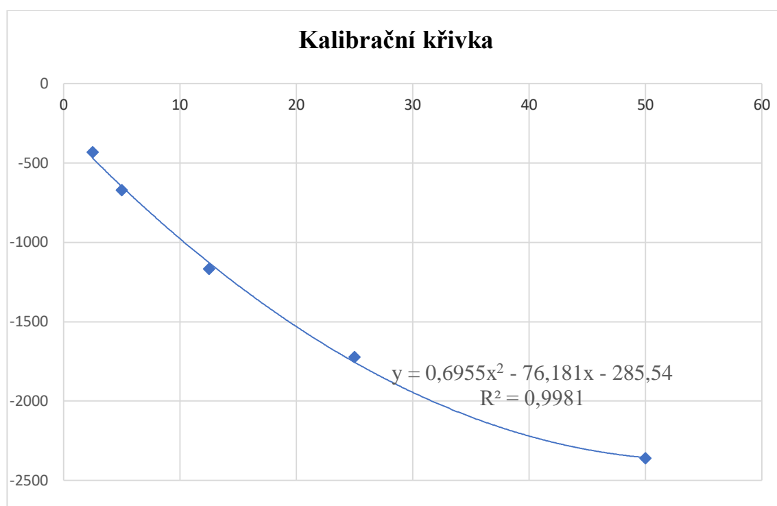
Obrázek 5- Kalibrační křivka
