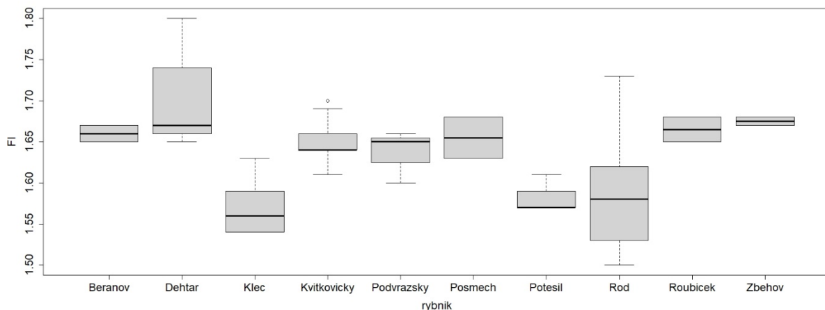
Obr. 19. Boxplot zobrazující hodnoty FI v jednotlivých rybnících (medián s kvartily a rozsahem minimálních a maximálních hodnot)
