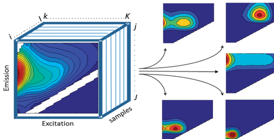
Obr. 7. Excitačně-emisní matrice rozložené do 5 komponentů PARAFAC (převzato z Murphy et al., 2013).
