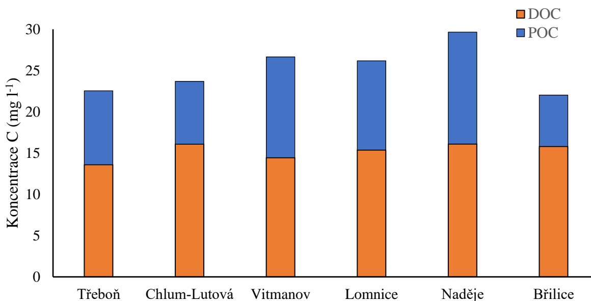
Obr. 12. Formy organického uhlíku DOC a POC v jednotlivých soustavách v letech 2010 – 2011. Sloupce zobrazují celkovou koncentraci TOC
