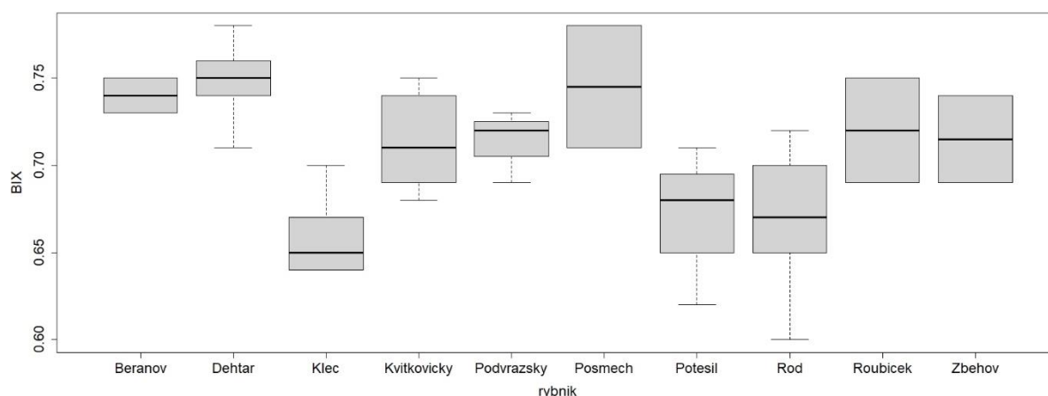
Obr. 20. Boxplot zobrazující hodnoty BIX v jednotlivých rybnících (medián s kvartily a rozsahem minimálních a maximálních hodnot)
