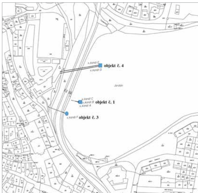
Obr. 2. Tábor – Jordán. Tři archeologicky zkoumané historické výpusti v hrázi. Čtverce – spodní výpusti, kolečko – horní výpust'. Čáry za čtverci a kolečkem naznačují směr odtékání vody mimo těleso hráze. Abb. 2. Tabor – Jordan-Stausee. Die drei archäologisch untersuchten historischen Ablässe im Damm. Quadrat – unterer Ablass, Kreis – oberer Ablass. Die Linien hinter den Quadraten und dem Kreis deuten den Verlauf der Abflussrichtung des Wasser außerhalb des Dammkörpers an.
