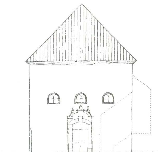
Zaměření Staré synagogy (příčný řez, čelní pohled), kresba Jaroslav Klenovský
