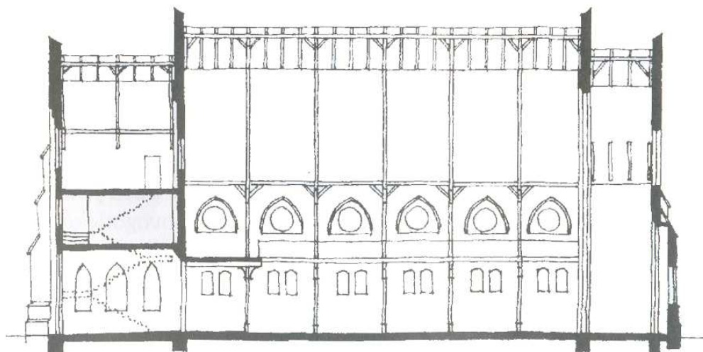
Zaměření Nové synagogy (podélný řez), kresba Jaroslav Klenovský
