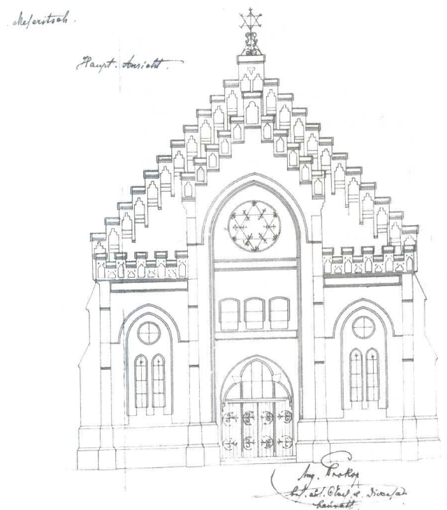
Originální návrh vstupního průčelí Nové synagogy, A. Prokop, 1868, ŽM Praha
