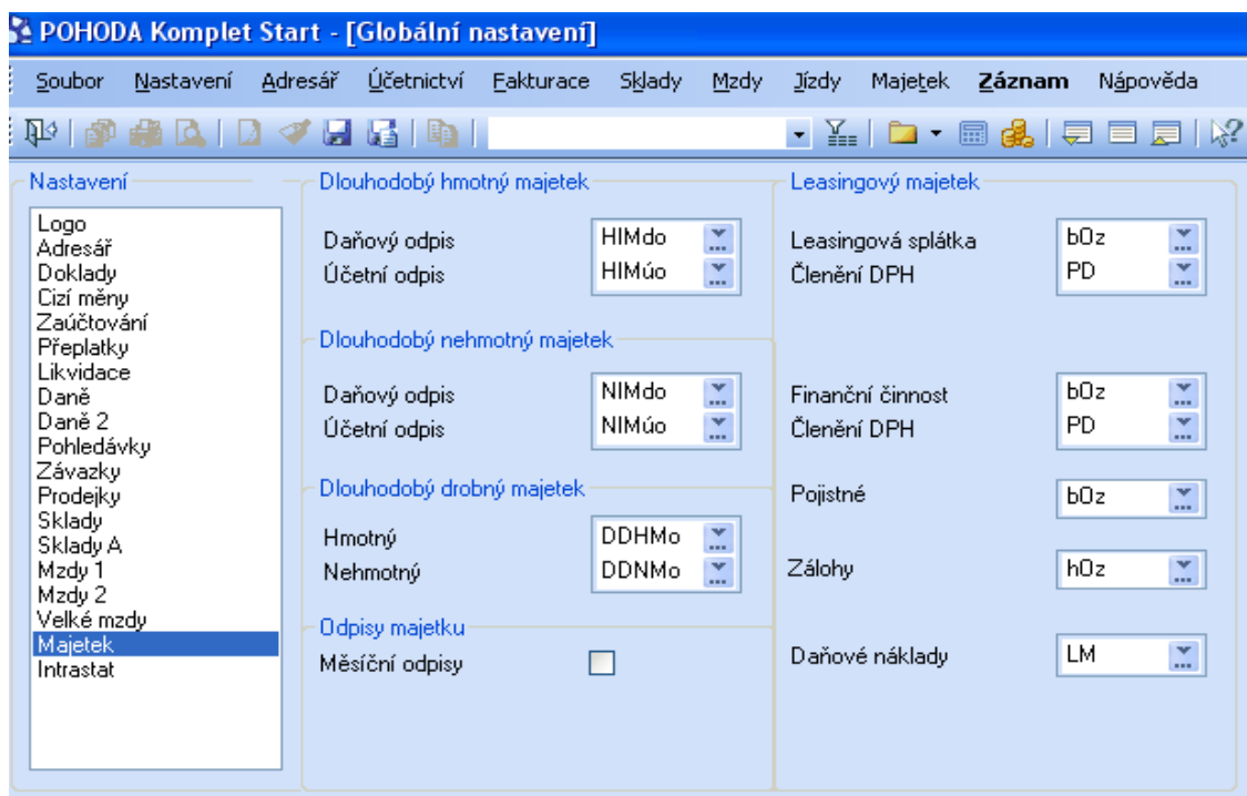
Obr. 9 Globální nastavení
