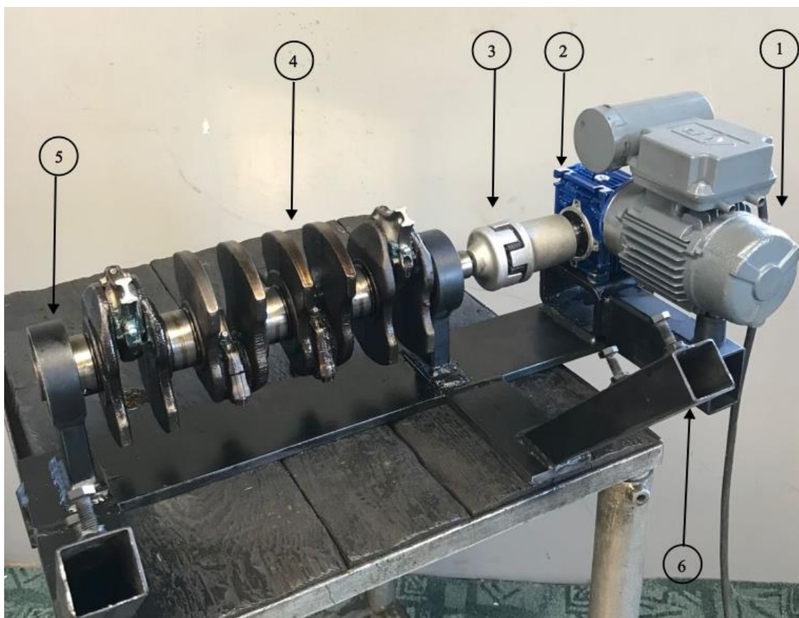
Obrázek č. 28: Testovací zařízení (1 – elektromotor, 2 – šneková převodovka, 3 – elastická spojka, 4 – kliková hřídel, 5 – ložiska, 6 – úchytná část).
