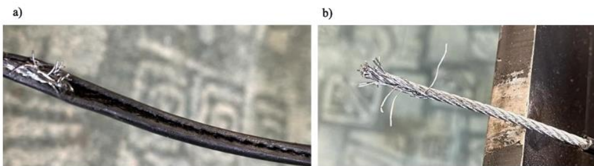
Obrázek č. 41: Přetržení poplastovaného lana – a) část s plastem, b) část bez plastu.
