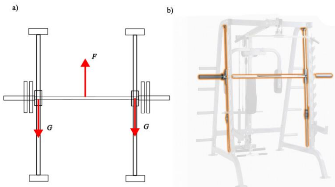
Obrázek č. 8: Multipress, část a) konstrukční schéma se značením působících sil, b) reálné vyobrazení stroje [20].
