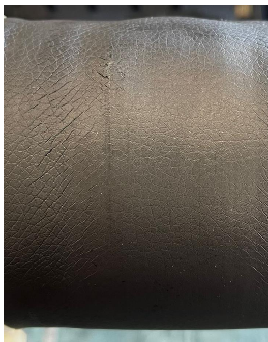
Obrázek č. 48: Otláčení eko kůže po provedení 10000 cyklů.
