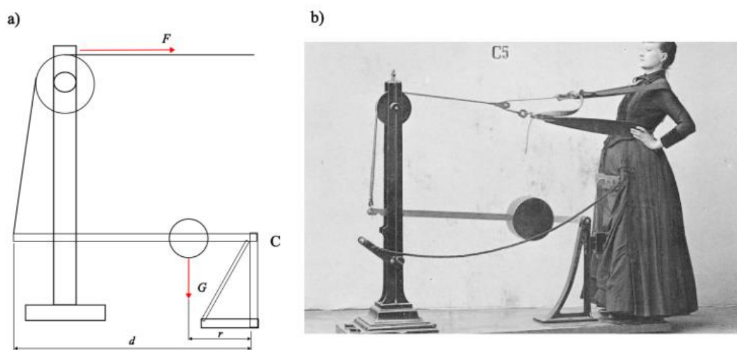
Obrázek č. 2: Historický posilovací stroj na svaly v oblasti zad, a) schéma konstrukčního provedení s naznačením působících sil, b) reálné vyobrazení stroje [3].
