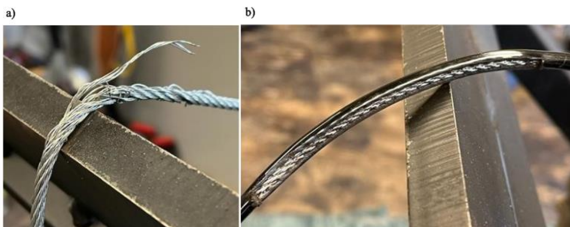
Obrázek č. 37: Kontrola po provedení 4720 cyklů – a) ocelové lano, b) ocelové lano poplastované.
