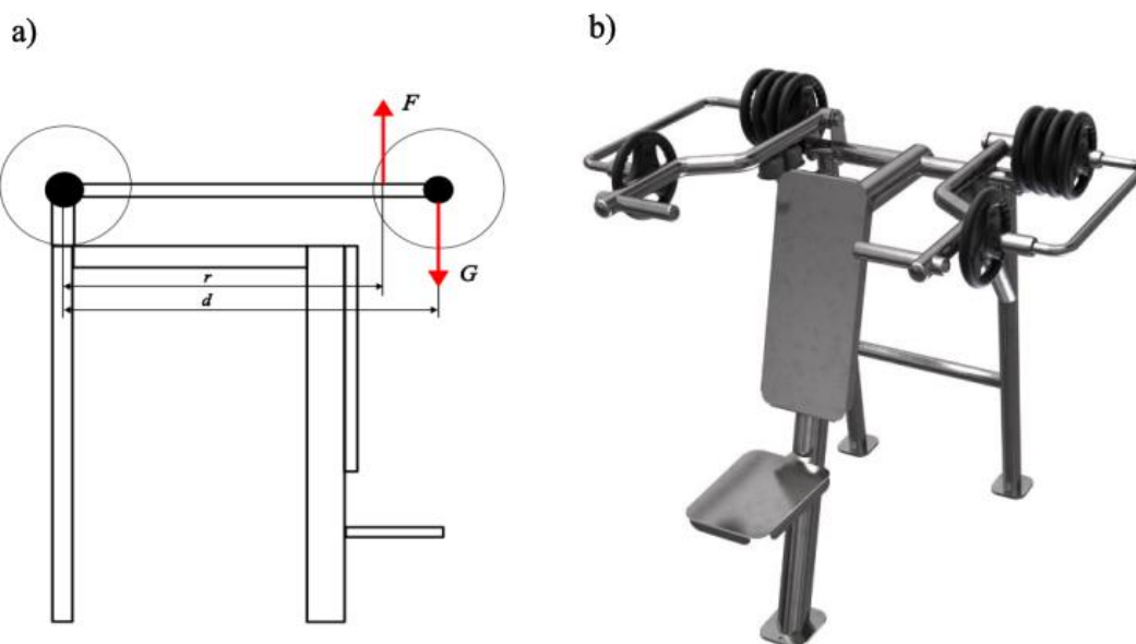
Obrázek č. 5: Shoulder press, část a) konstrukční schéma se zaznačením působících sil, b) reálné vyobrazení stroje [17].
