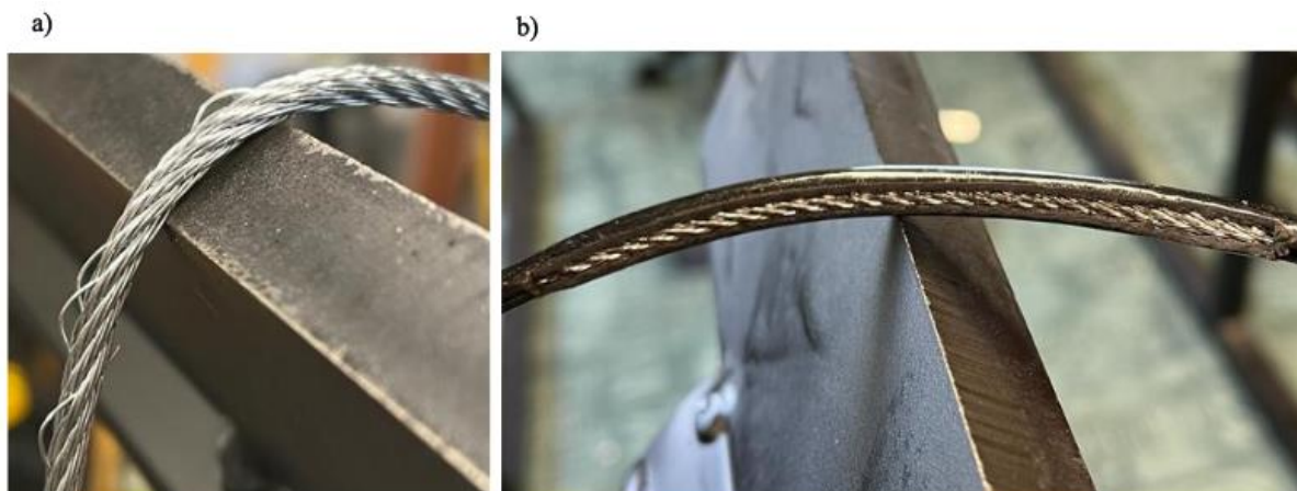
Obrázek č. 34: Kontrola po provedení 1520 cyklů – a) ocelové lano, b) ocelové lano poplastované.
