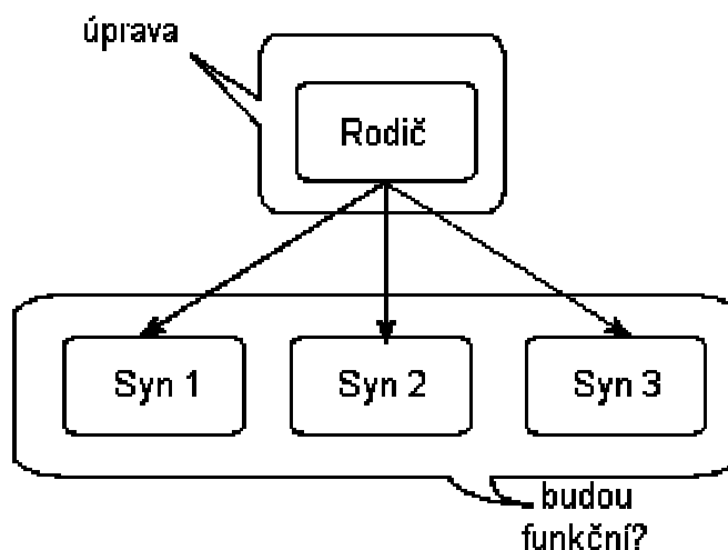
Obr. 4: úprava tříd
