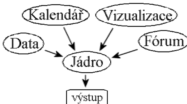
Obr. 3: distribuovaný systém
