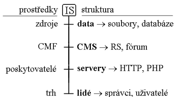
Obr. 1: informační systém
