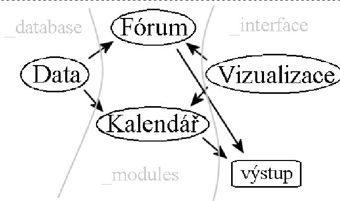
Obr. 3: distribuovaný systém
