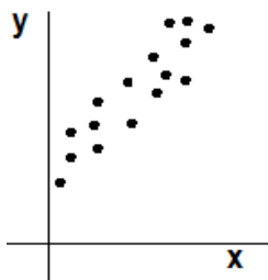
Obr. 2 - Graf silné přímé lineární závislosti (Popjaková 2013)
