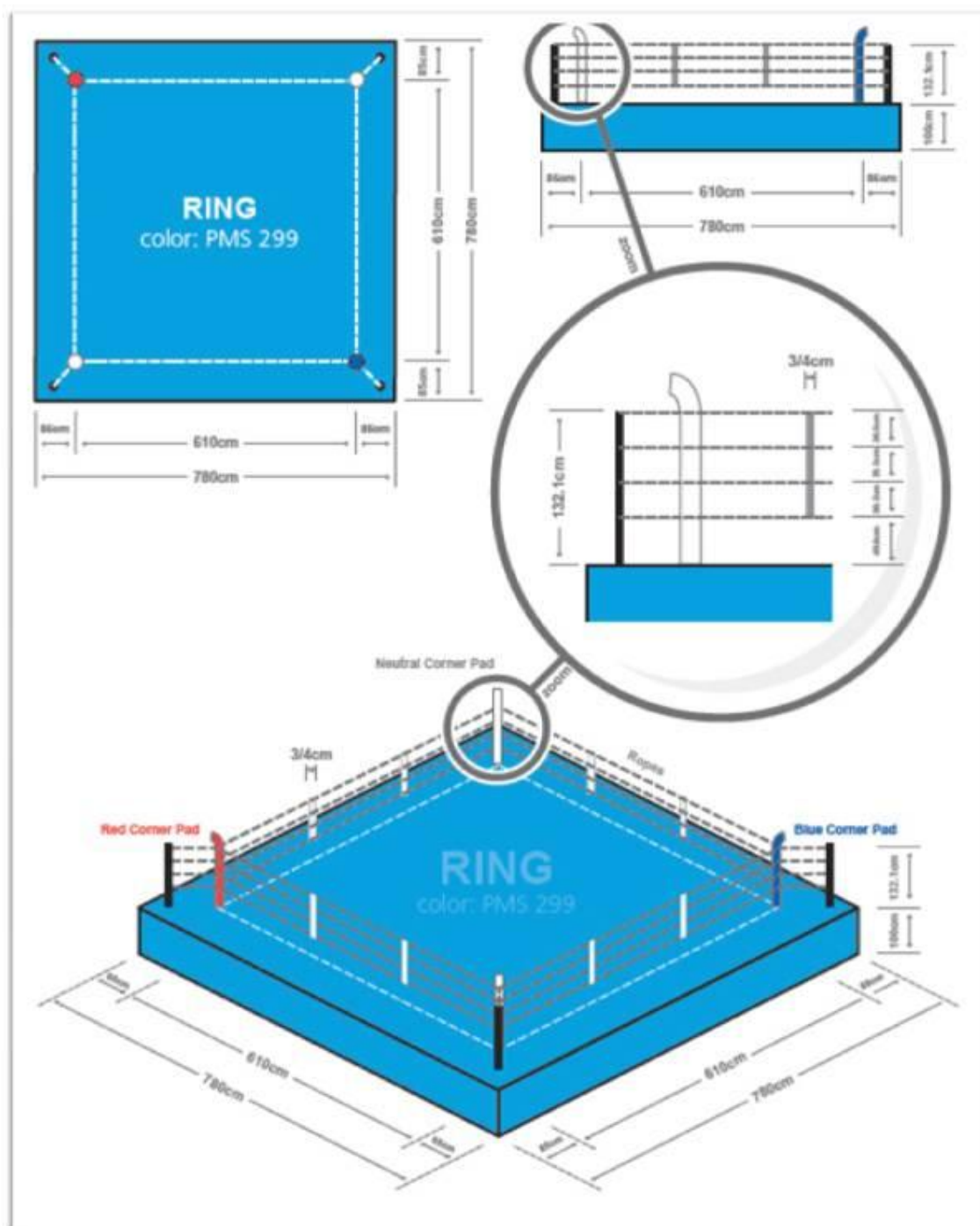
Obrázek 1. Rozměry ringu podle pravidel AIBA.
